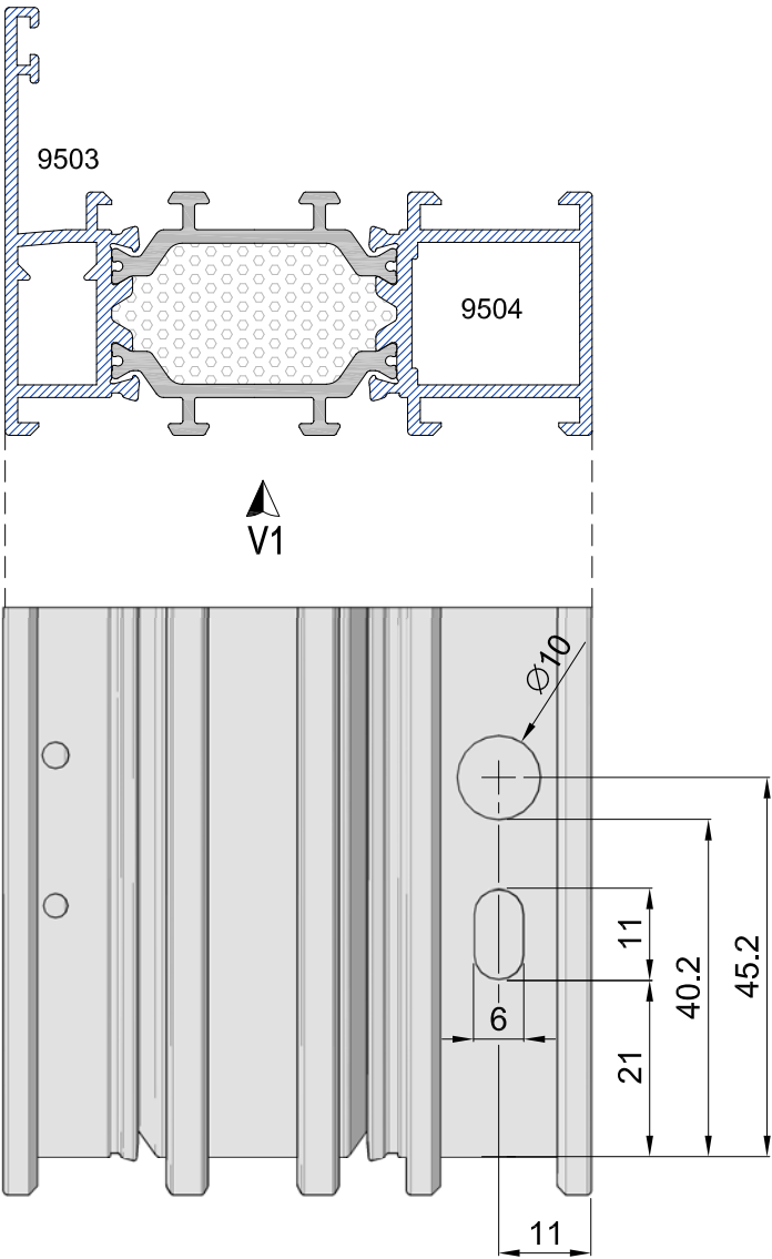
Mecanizado escuadra A495467B V1 M4 1:1
