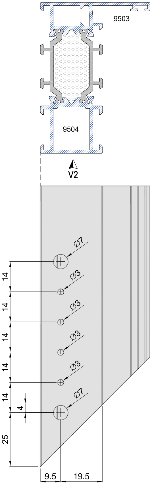
Mecanizado bisagra MACO M9 (posición intercambiable)
