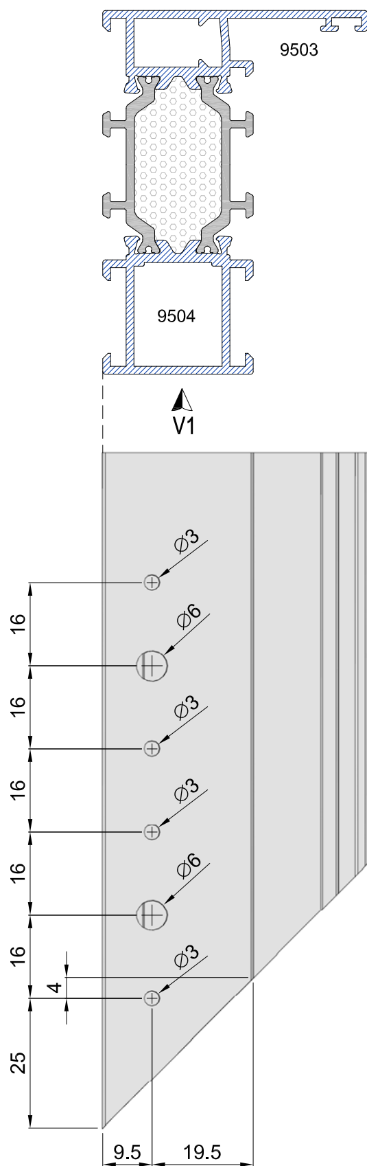
Mecanizado bisagra ROTO M9 (posición intercambiable)
