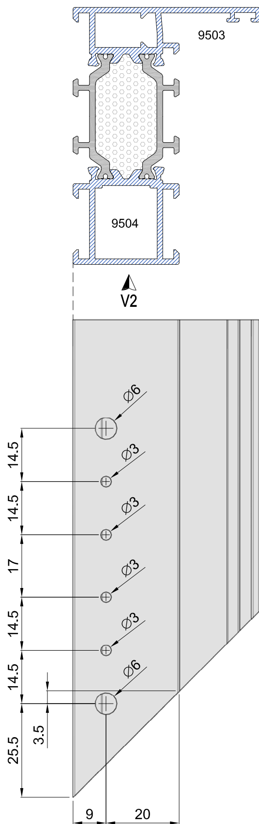
Mecanizado bisagra VBH M9 (posición intercambiable)
