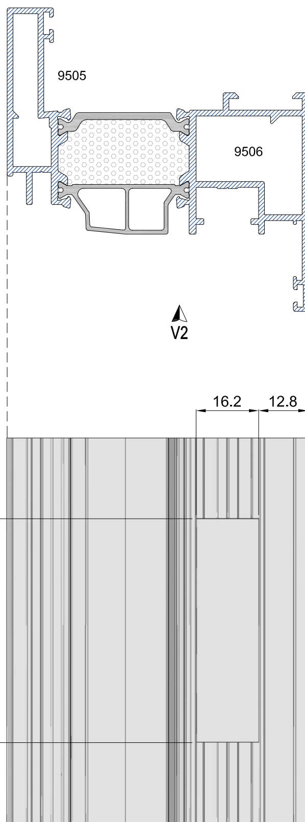
Mecanizado cajera cremona M6
