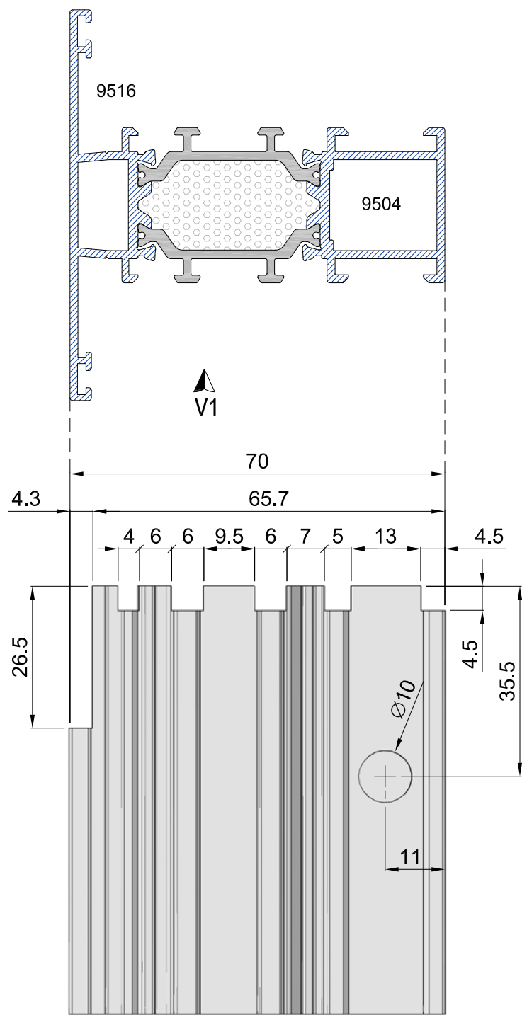
Mecanizado del tope zanca M5 ( solo hace el taladro ) V1 1:1
