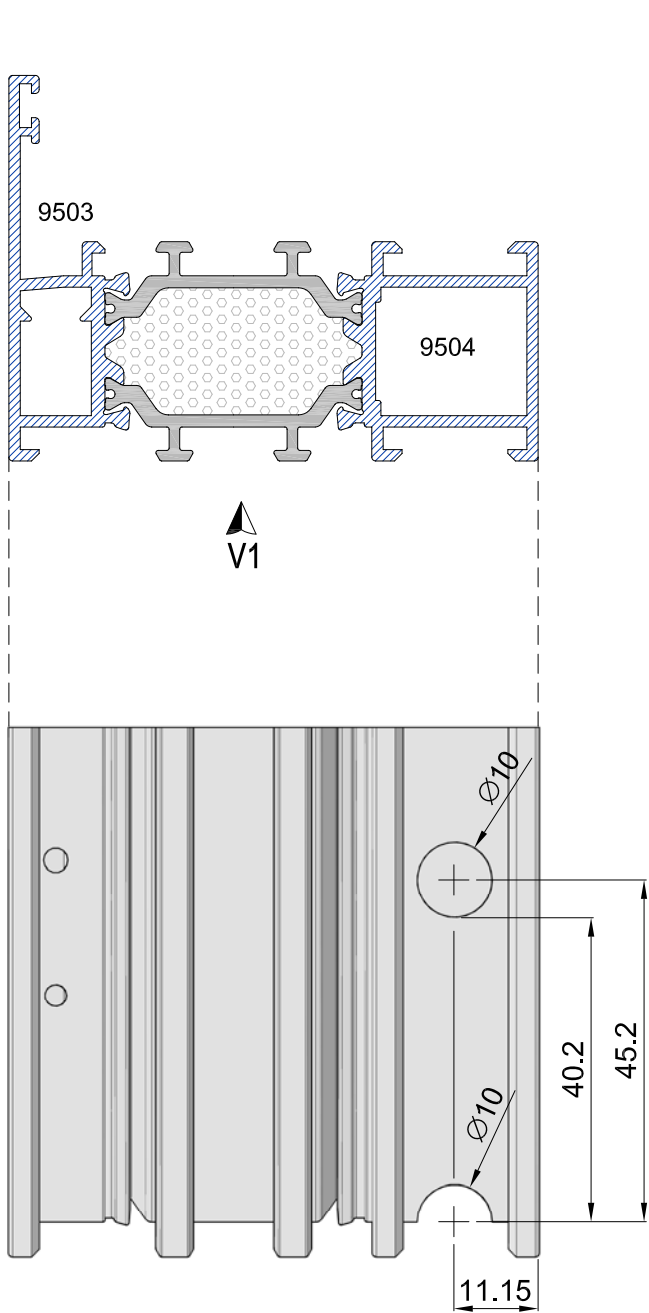
Mecanizado escuadra A495346B Opcional
