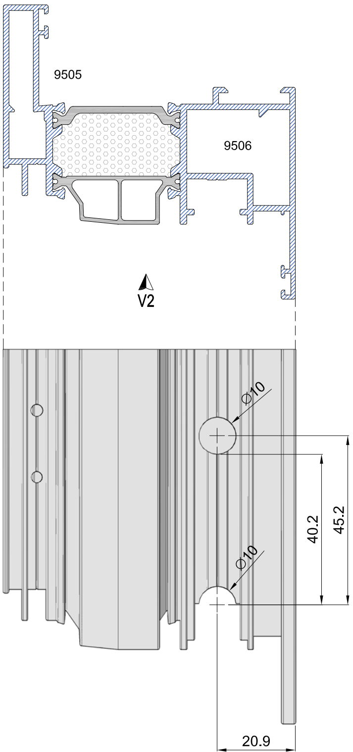
Mecanizado escuadra A495346B Opcional
