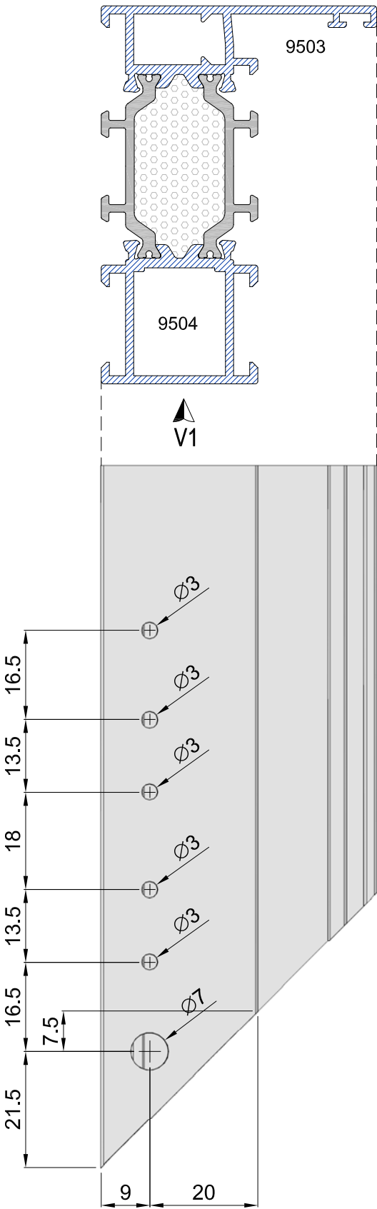
Mecanizado bisagra FUHR M9 (posición intercambiable)
